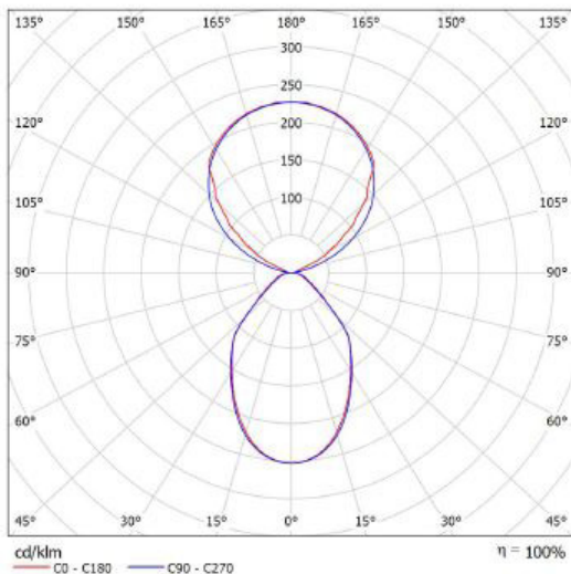
Lichtverteilungskurve HXL-Fuss 4000K asymmetrisch (LVK)
