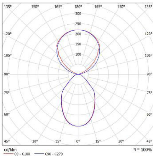
Lichtverteilungskurve U-Fuss 4000K asymmetrisch (LVK)
